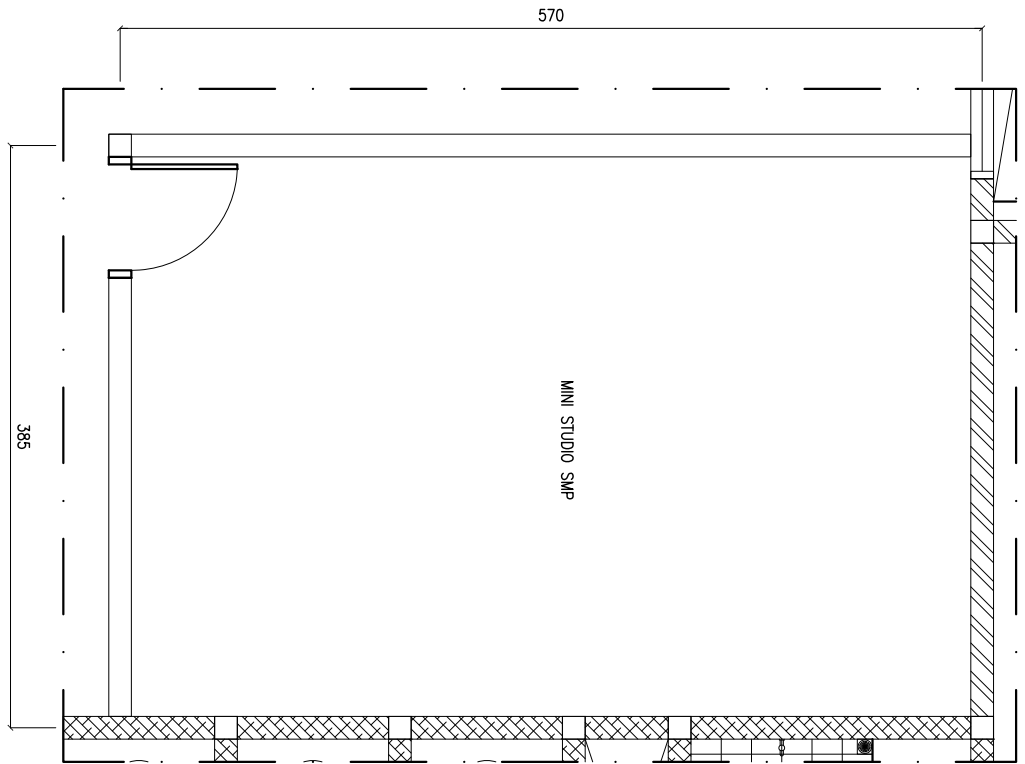
DENAH EKSTING MINI STUDIO SMP SKALA 1 : 50
